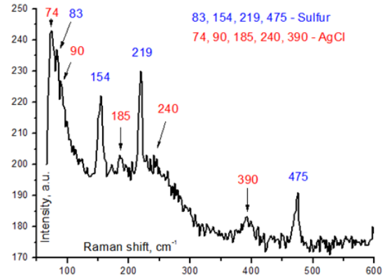
Рис. 2. КР спектры образца S–AgCl: идентификация пиков серы и AgCl.
