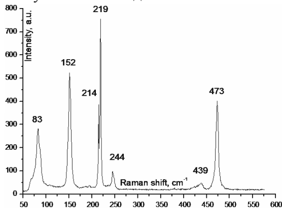
Рис. 3. Идентификация КР спектров S–AgCl–Ag 2 S.
