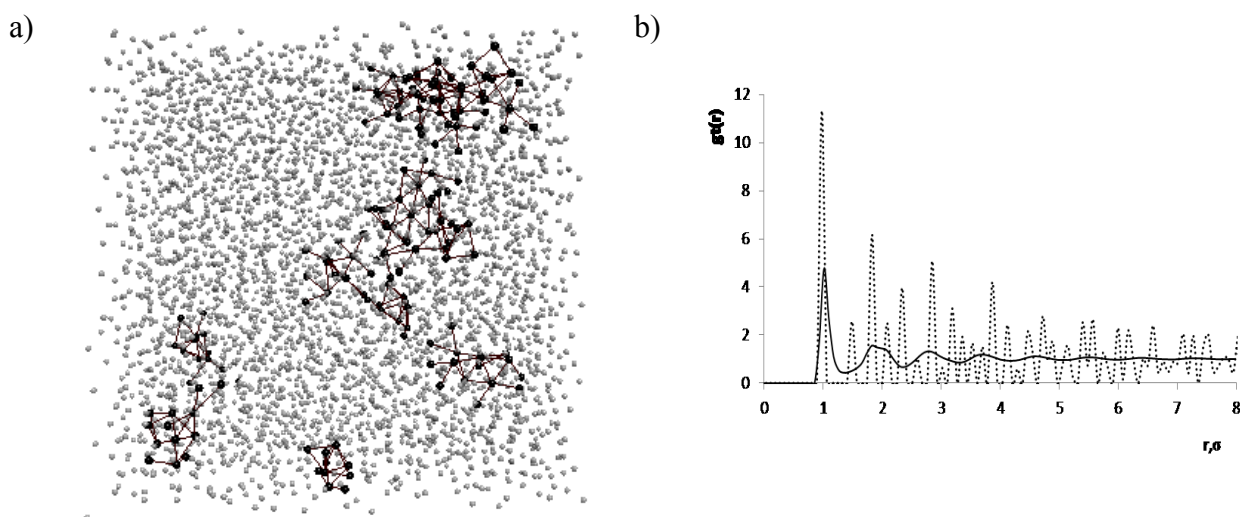
Рис. 3. Конфигурация частиц аргона (а) и радиальная функции системы (б), полученной в результате охлаждения со скоростью 10^{10} К/с
