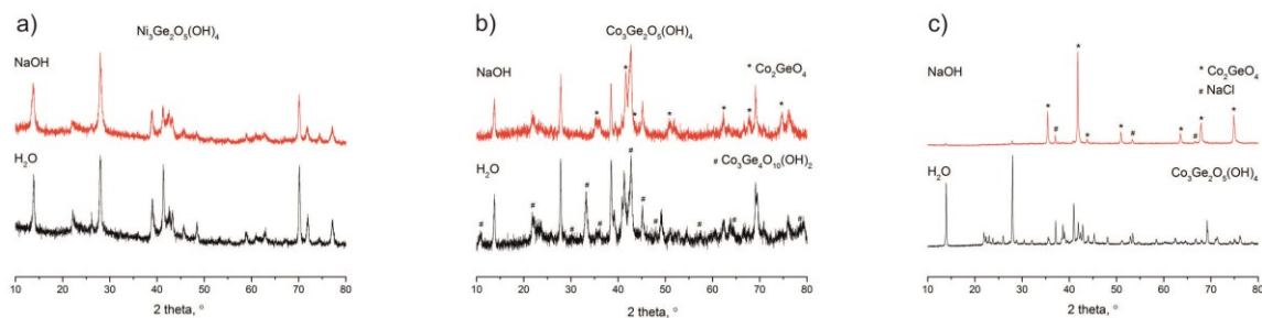
Рисунок 1 – Дифрактограммы полученных образцов: а) гидрогерманаты никеля; б) гидрогерманаты кобальта, синтезированные на воздухе; в) гидрогерманаты кобальта, синтезированные в атмосфере аргона.
