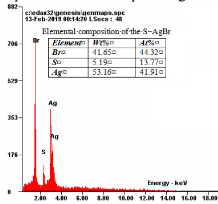
Рис. 4. Элементный состав S–AgBr.
