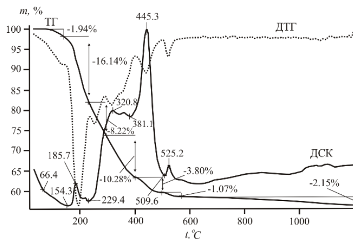
Рис. 2. Термический анализ танталсодержащего остатка с примесью гадолиния,
