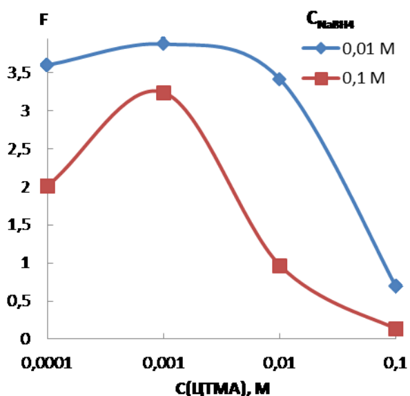
Рис. 2. Зависимость функции Кубелки-Мунка нанокompозита от концентрации ЦТМА в растворе.
