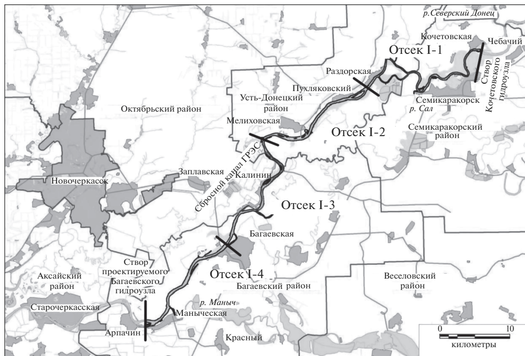
Рис. 1. Картограмма Багаевского водохранилища с делением на расчетные отсеки.
