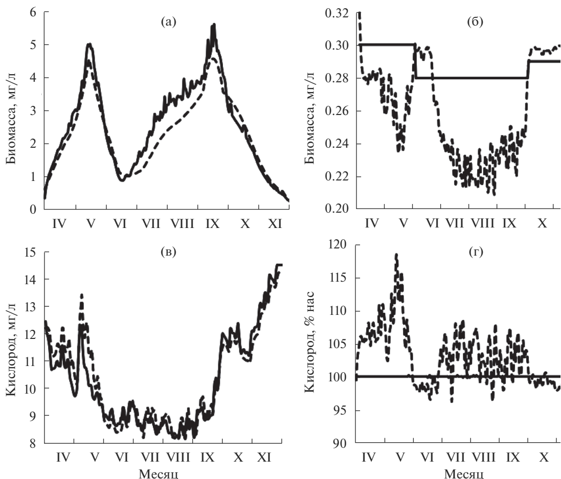
Рис. 2. Поступающие в водохранилище (сплошная линия) и рассчитанные по модели (пунктирная линия) изменения биомассы фитопланктона (а), суммы минеральных форм азота и фосфора (б), содержание кислорода (в) и насыщение воды (г) растворенным кислородом в отсеке 1-4 в 1986 г.
