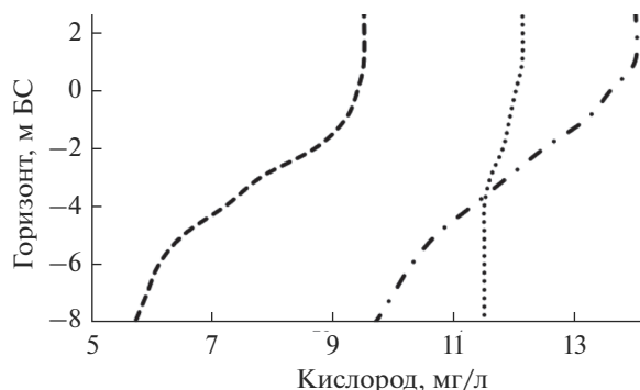
Рис. 4. Рассчитанное вертикальное распределение содержания кислорода на приплотинном участке (отсек I-4) водохранилища при проектном НПУ 2.8 м на 15 апреля (сплошная линия), 15 мая (штрихпунктирная линия), 15 августа (пунктирная линия) и 15 октября (точки).
