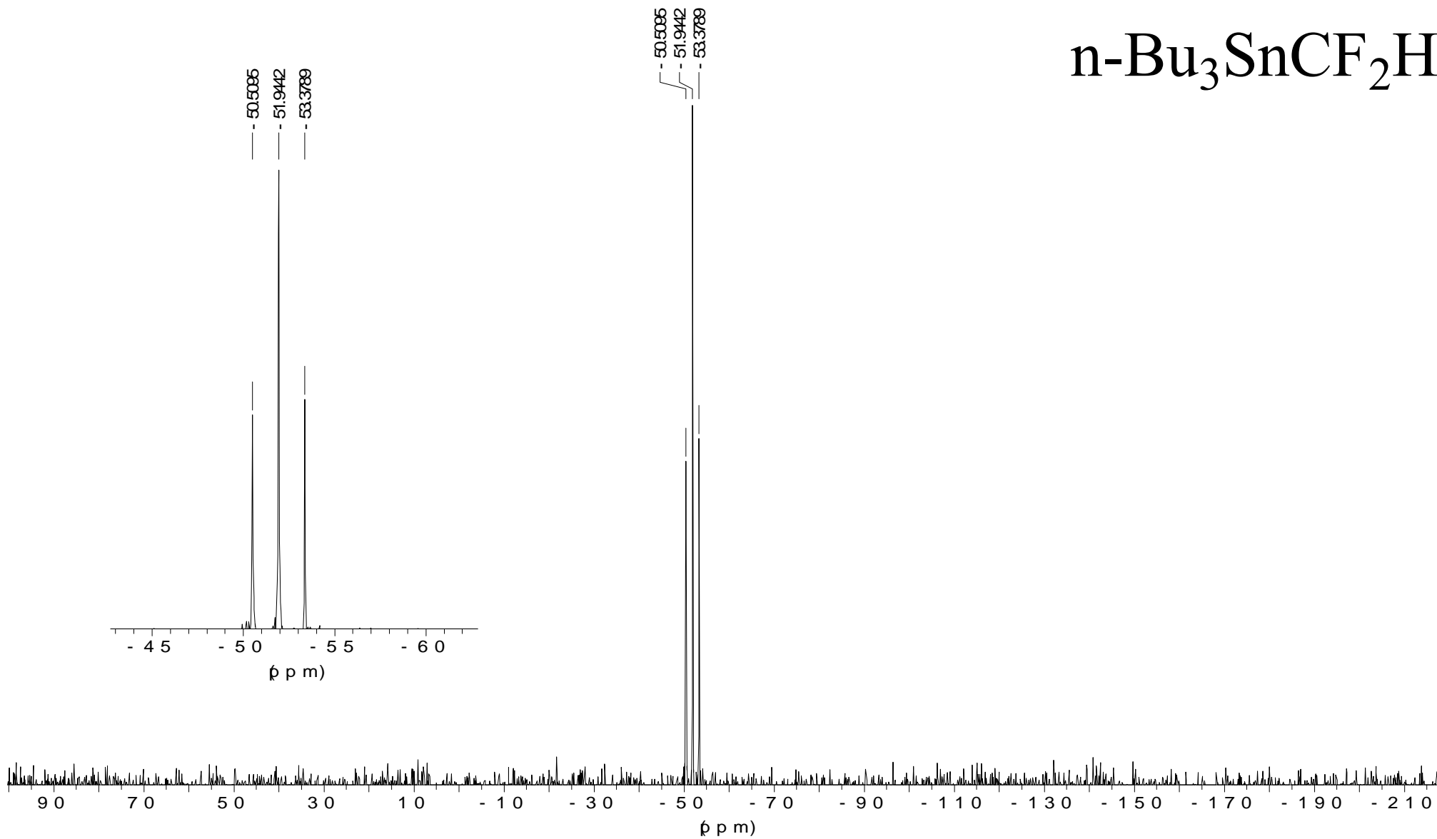
Спектр ЯМР ^{119}\text{Sn} (дифторметил)трибутилстаннана в \text{CDCl}_3
