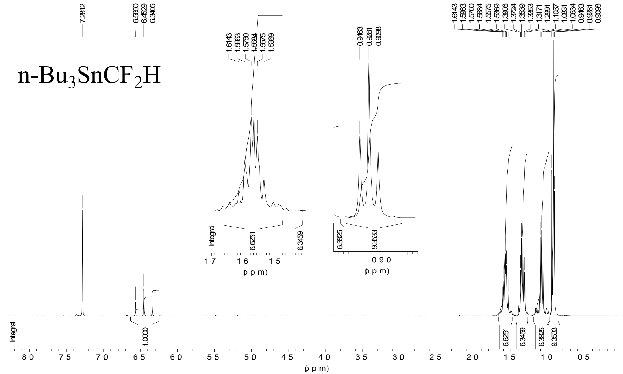
Спектр ЯМР ^1\text{H} (диформетил)трибутилстаннана в \text{CDCl}_3
