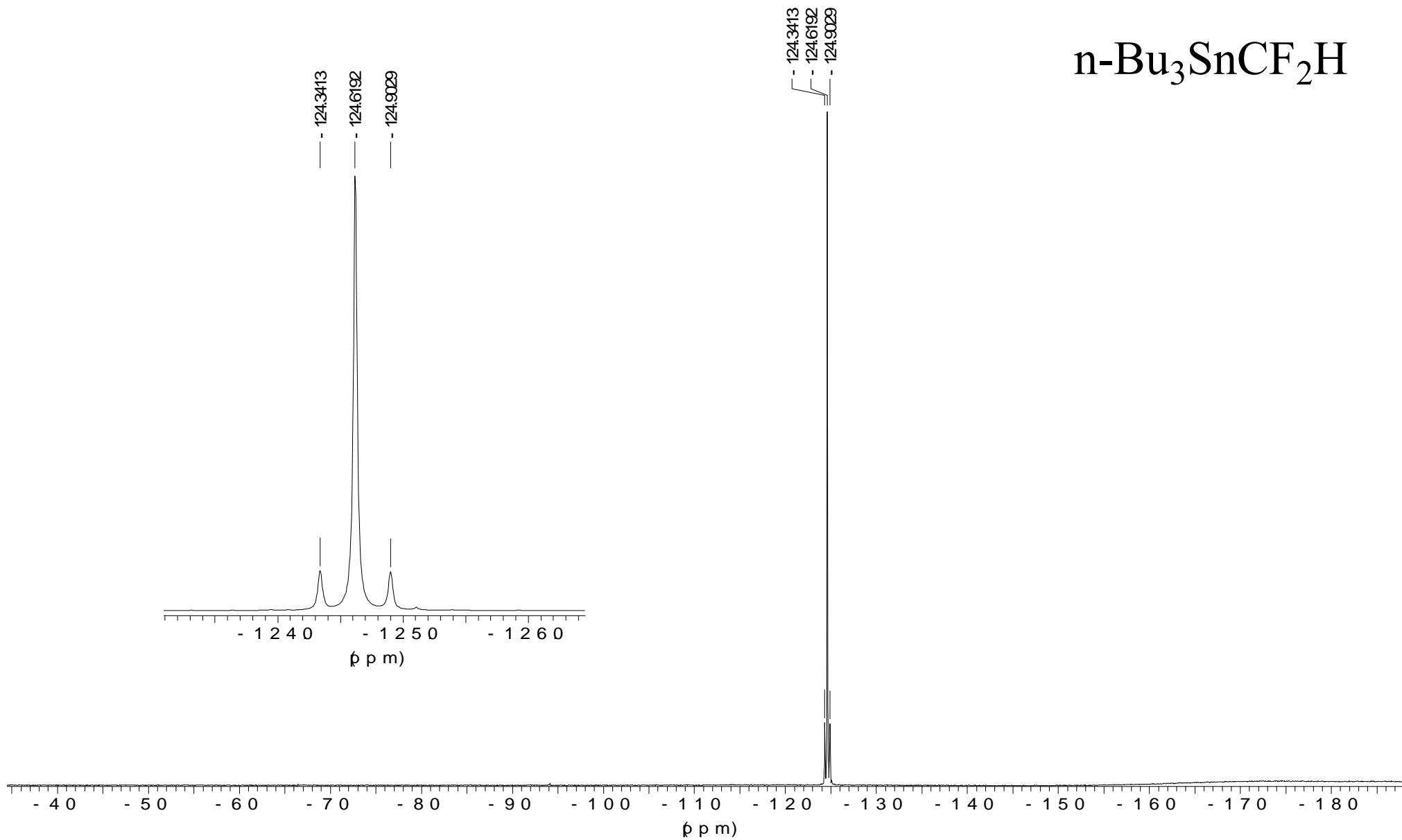
Спектр ЯМР ^{19}\text{F}\{\text{H}\} (дифторметил)трибутилстаннана в \text{CDCl}_3
