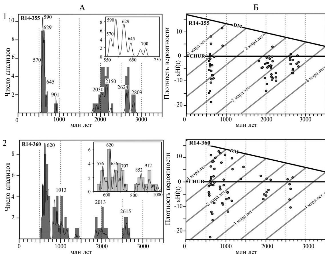
Рис. 5. Гистограммы и графики плотности вероятности распределения возрастов детритовых цирконов с детализацией для интервалов 500–1000 млн лет (А) и диаграмма \epsilon_{\text{Hf}} - \text{возраст} (Б) для детритовых цирконов из ордовикских песчаников Зауральской мегазоны (пробы R14-355-1и R14-360).
