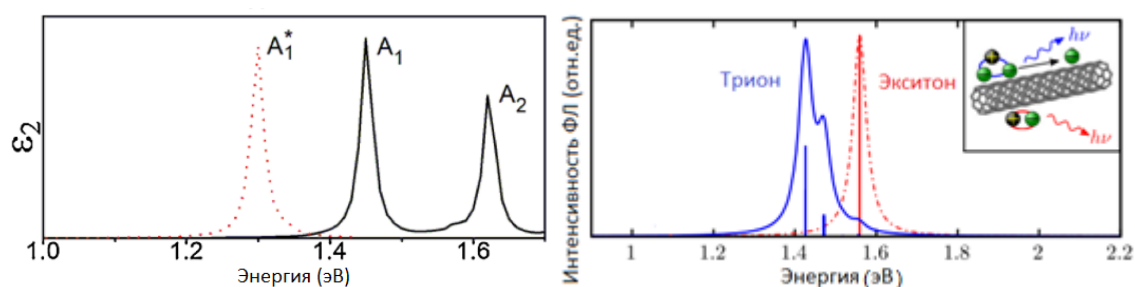
Рис. 16 а) Теоретический расчет энергии свободных экситонов ( A_1 и A_2 ) и экситонов, локализованных на дефекте в (8,0) -ОУНТ при допировании кислородом ( A_1^* ). [129] б) Теоретический расчет энергии экситонов и трионов в (8,0) -ОУНТ при n -допировании [132]
