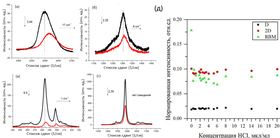
Рис. 53(а-г) Спектры КРС в исходных (черная линия) и допированных ОУНТ при концентрации HCl 2 мкл/мл. Длина волны возбуждения 633 нм. д) Зависимость отношения интенсивностей различных мод КРС к интенсивности тангенциальной моды.
