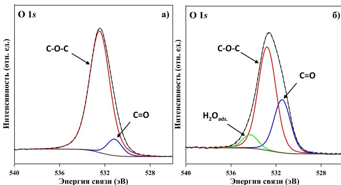
Рис. 21. О 1s РФЭ-спектры высокого разрешения образцов №23 (а) и №22 (б).
