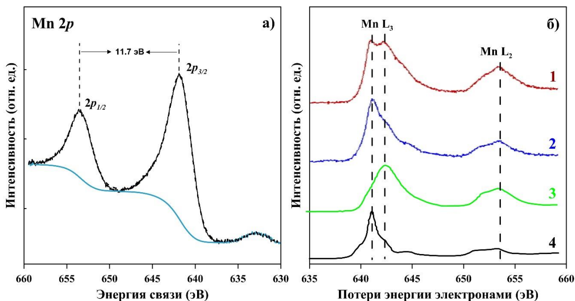
Рис. 39. Mn 2p РФЭ-спектр высокого разрешения нанокompозита №60 (а); спектры EELS с различных областей образца №60 (б), соответствующие литературным данным для Mn 3 O 4 (1) и MnO (2), спектры стандартов Mn 2 O 3 (3) и MnO (4) [270].
