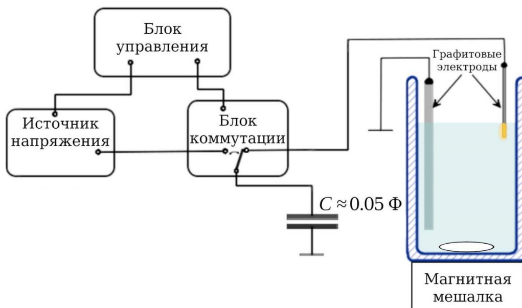
Рис. 12. Блок-схема установки.
