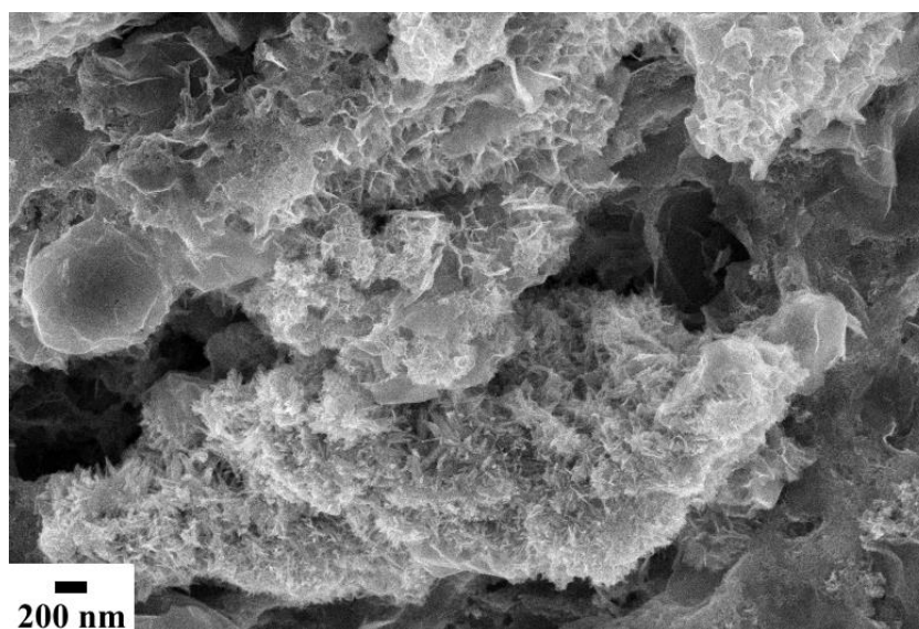
Рис. 37. СЭМ-изображение нанокompозита №60.
