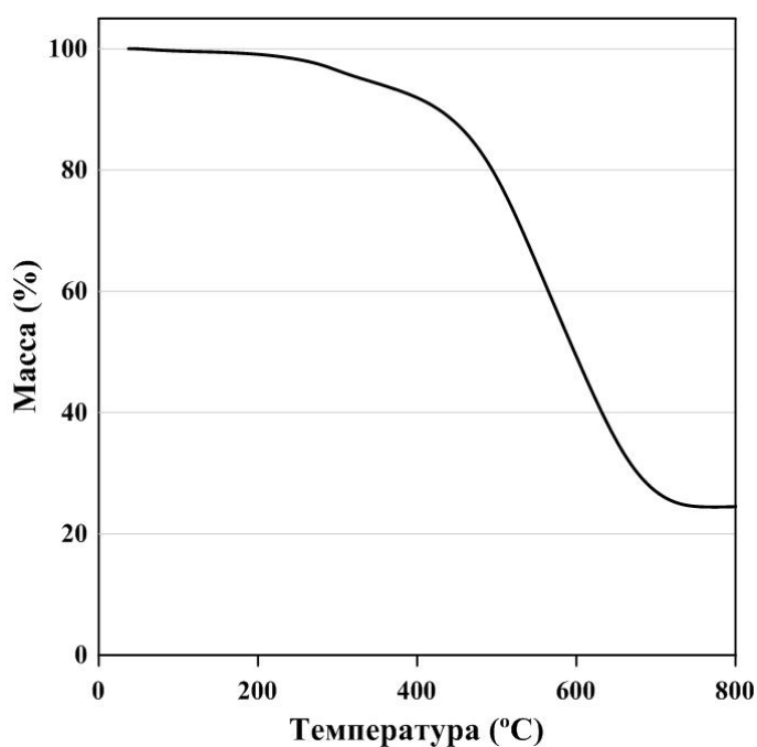
Рис. 46. ТГА-зависимость нанокompозита №80.
