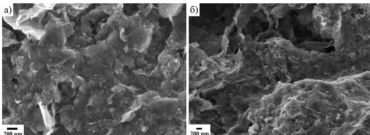
Рис. 45. СЭМ-изображения нанокompозитов №78 (а) и №79 (б)
