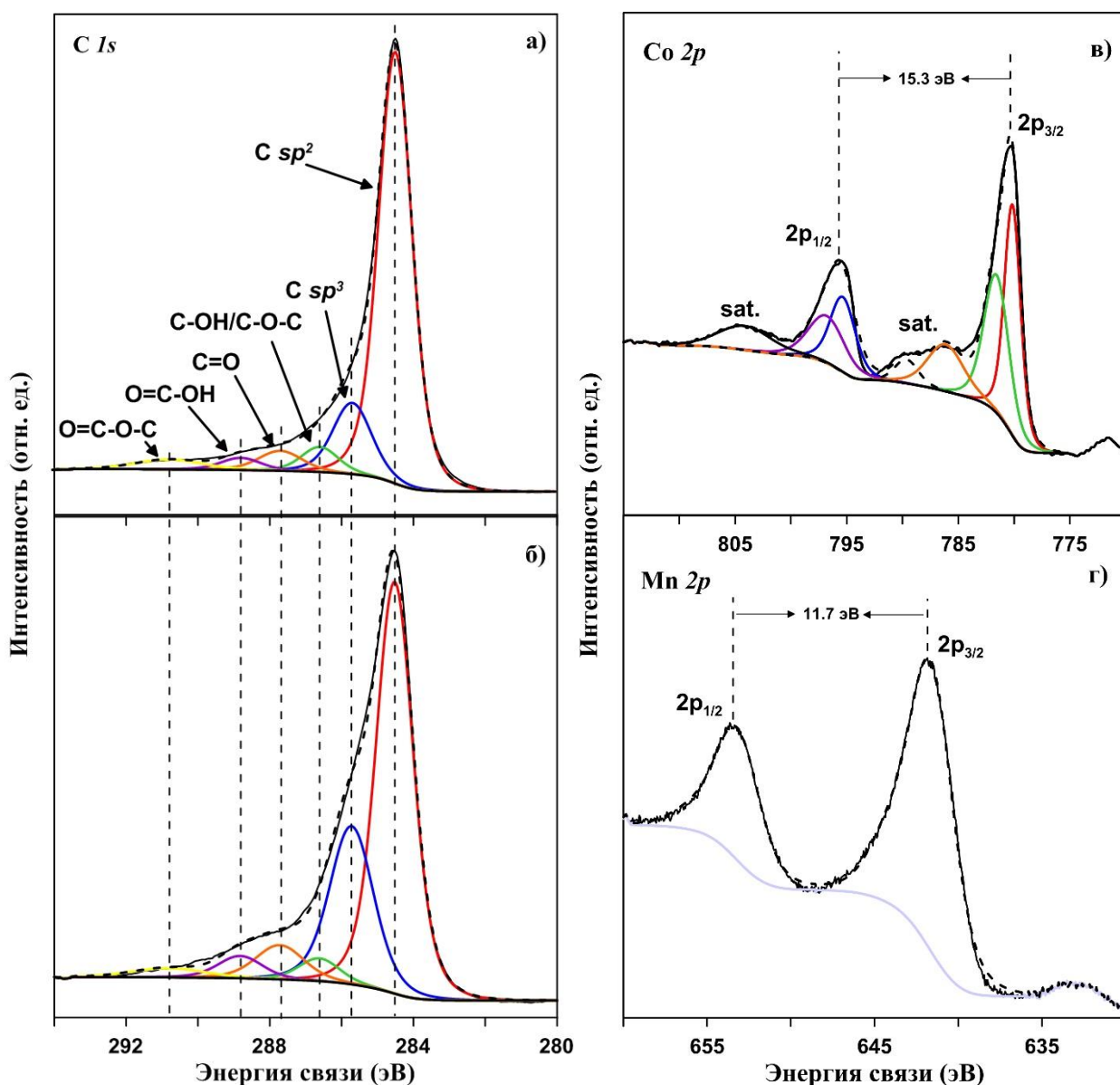
Рис. 48. РФЭ-спектры высокого разрешения C 1s, Co 2p и Mn 2p нанокomпозитов №78 (а,в) и №79 (б,г).
