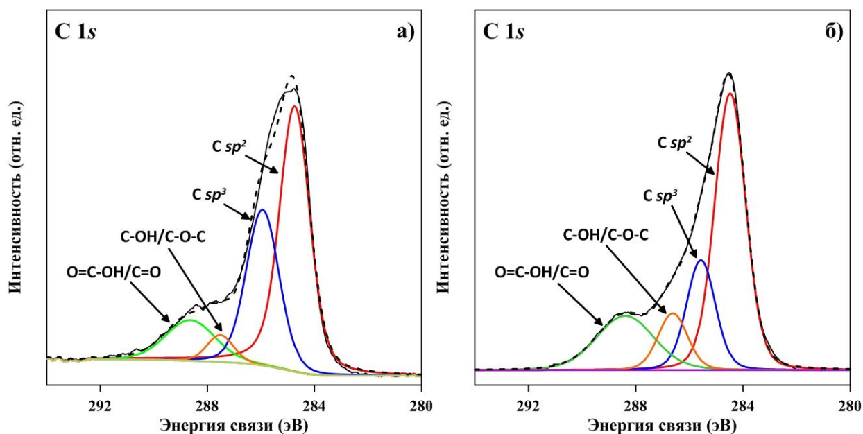
Рис. 68. C 1s РФЭ-спектры высокого разрешения наноккомпозитов №170 (а) и №180 (б).
