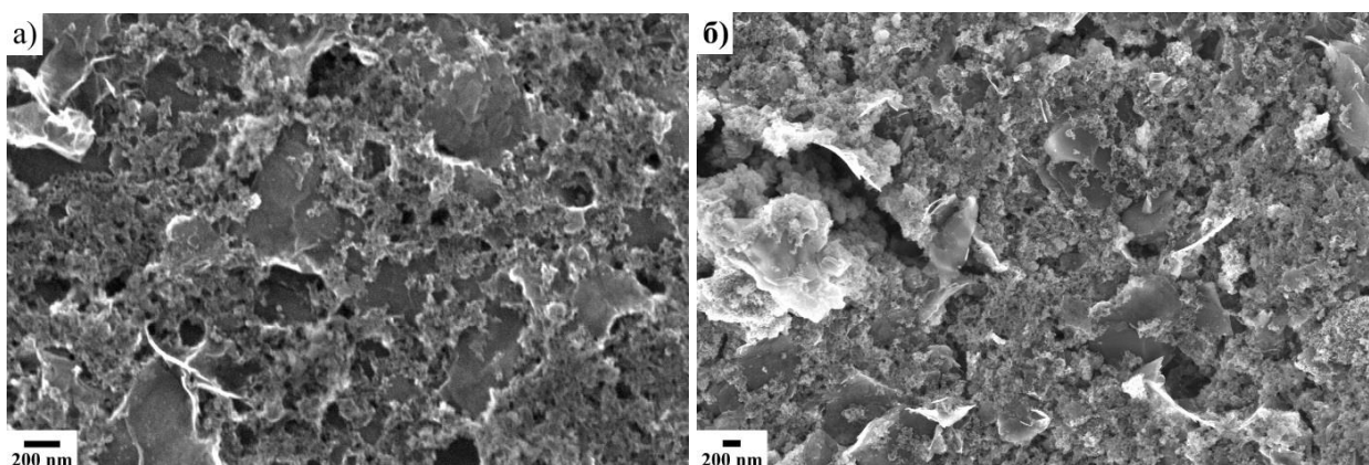
Рис. 66. СЭМ-изображения наноконкомпозитов №170 (а) и №180 (б).
