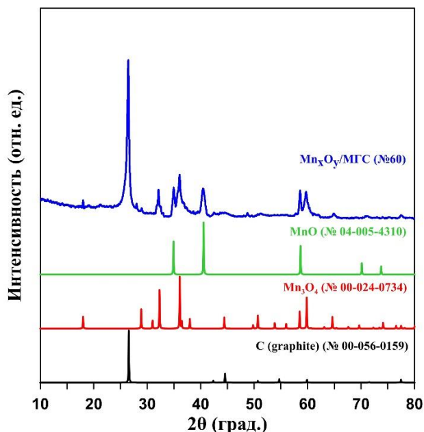
Рис. 38. Рентгенограмма нанокompозита №60.
