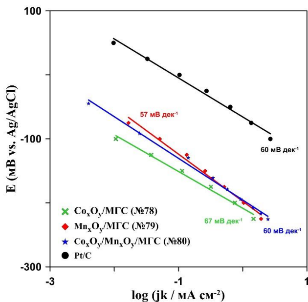
Рис. 50. j, E -зависимости образцов №78–80 в координатах Тафеля.
