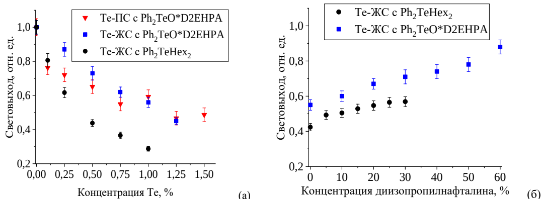
Зависимость световыхода теллурсодержащих органических сцинтилляторов от концентрации (а) теллура, (б) диизопропилнафталена (относительно световыхода образцов ЖС или ПС, не содержащих теллур)
