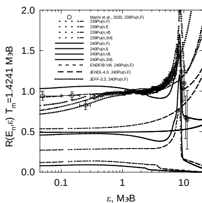
Рис. 1 СМНД ^{239,240}\text{Pu}(n,F)
