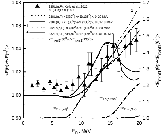
Рис. 2. ^{232}\text{Th}(n, F) и ^{238}\text{U}(n, F) , отношения \langle E \rangle , \langle E_{n,xf} \rangle для 30^\circ/135^\circ
