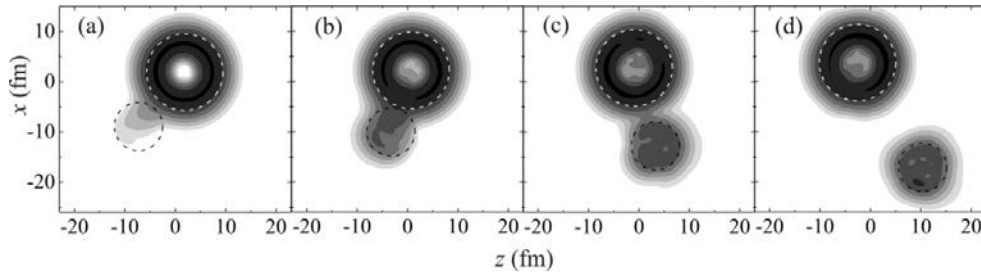
Рис. Пример временной эволюции плотности вероятности (оттенки серого, логарифмическая шкала) для протона подболочки 1h_{1/2} ядра ^{197}\text{Au} в столкновении ^{48}\text{Ca} + ^{197}\text{Au} при энергии в системе центра масс 400 МэВ и прицельном параметре 9 фм. Расположение панелей (a)–(d) соответствует времени
