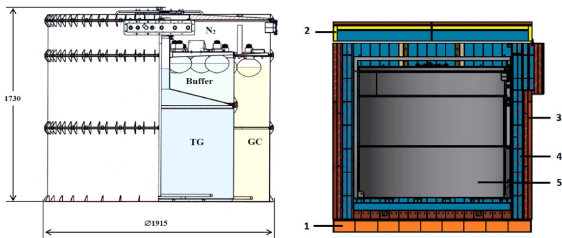
Рис. Слева: детектор имеет 3 объема – буфер (заполненный чистым ЛАБом), мишень (заполненную гадолиниево-содержащим сцинтиллятором), гамма-кетчер (заполненный сцинтиллятором). Справа: 1 – чугун, 2 – свинец, 3 – чистый полиэтилен, 4 – борированный полиэтилен, 5 – детектор
