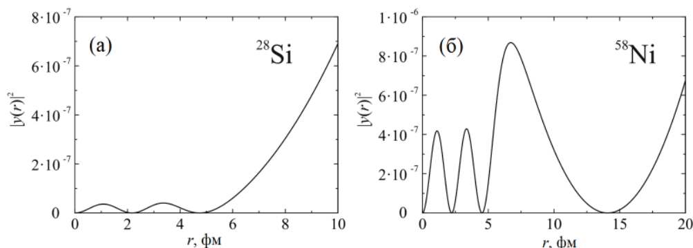
Рис. Радиальные плотности вероятностей s -состояний медленных нейтронов при упругом рассеянии на ядрах ^{28}\text{Si} (а) и ^{58}\text{Ni} (б).
