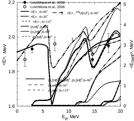
Рис. 1. \langle E \rangle и \langle E_{n,xf} \rangle для ^{232}\text{Th}(n, F) и ^{238}\text{U}(n, F)
