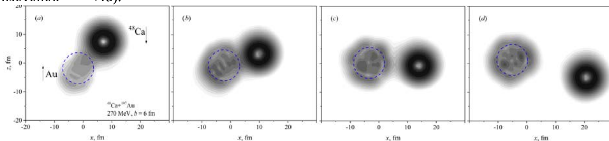
Эволюция плотности вероятности нейтрона 1f_{7/2} -ядра ^{48}\text{Ca} при касательном столкновении ядер ^{48}\text{Ca} + ^{197}\text{Au} . Энергия 270 МэВ, прицельный параметр b = 6 фм. Ход времени соответствует направлению слева направо
