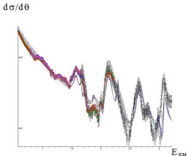
Рисунок. Функция возбуждения реакции ^{16}\text{O}(d,d_0) под углами 153.6 – 169.2 градусов в с.ц.м (точки – экспериментальные значения, сплошные кривые – описание).
