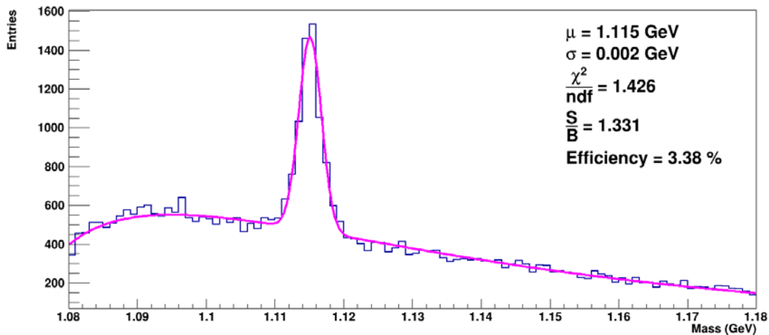
Рис. 1. Распределение по инвариантной массе пар протон — отрицательный пи-мезон. Фиолетовым цветом показана аппроксимация пика лямбда-гиперонов и фона суммой гауссовой функции и произведения радикальной функции и экспоненты.
