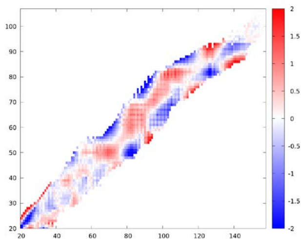
Отклонение в МэВ значений масс ядер, рассчитанных на основе разностного соотношения \Delta_{\text{пр}} , от данных AME2020.
