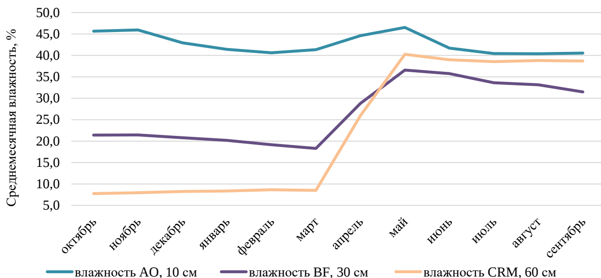
Рисунок 3. График среднemesячных значений годового распределения влаги в органокриометаморфической почве Аганского увала
