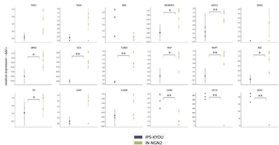
Рисунок 7. Уровни относительной экспрессии маркерных генов, определенные методом количественной ОТ-ПЦР в 17-дневных нейральных культурах iN-NGN2. По оси Y показан уровень экспрессии, рассчитанный методом -\Delta\Delta Ct , нормализованный к экспрессии генов домашнего хозяйства ( EMC7 и PSMB4 ). Каждая точка представляет собой биологическую реплику. Столбики ошибок указывают на стандартное отклонение технических реплик. Звездочки указывают на статистическую значимость различий, рассчитанную с помощью теста Уэлча (* – p-value <0,05, ** – p-value <0,01).
