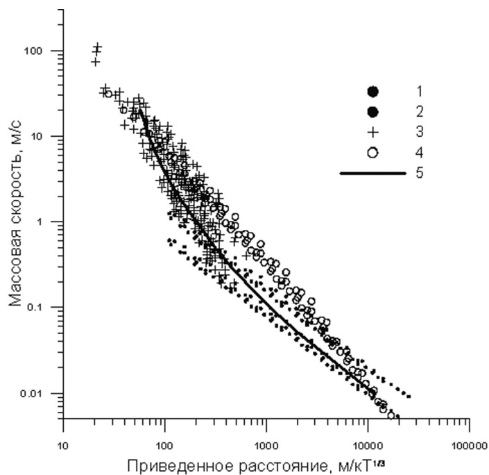
Рис. 11. Зависимости величин массовых скоростей от приведенного расстояния для взрывов и землетрясений. 1, 2 – характерные пределы зависимости для землетрясений по данным табл. 2; 3 – данные по взрывам на скальной площадке «Дегелен» Семипалатинского полигона (по [Kocharyan, Spivak, 2003]); 4 – характерные максимальные значения для землетрясений, по табл. 5; 5 – характерная общая тенденция изменчивости по данным (1–3).
