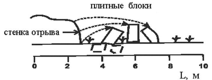
Рис. 5. Вариант скола блоков от стенки массива в соответствии с моделью № 1.
