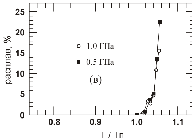
Рис. 4 Зависимость удельного сопротивления (а), скорости продольных волн (б) и содержания расплава (в) от гомологической температуры
