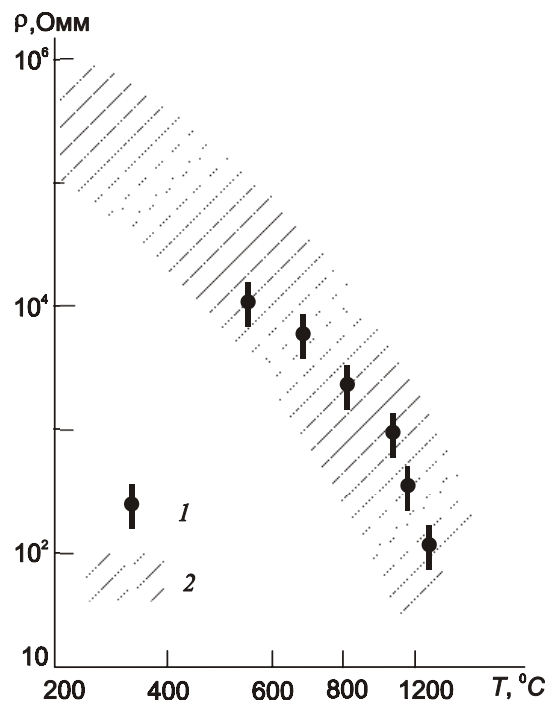
Рис. 1 Зависимость удельного электрического сопротивления ультраосновных пород от температуры: 1 – данные С.С.Реем и М.Г.Маньяни; 2 – область экспериментальных результатов различных авторов
