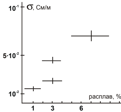
Рис. 5 Зависимость электропроводности ультраосновных пород от содержания расплава
