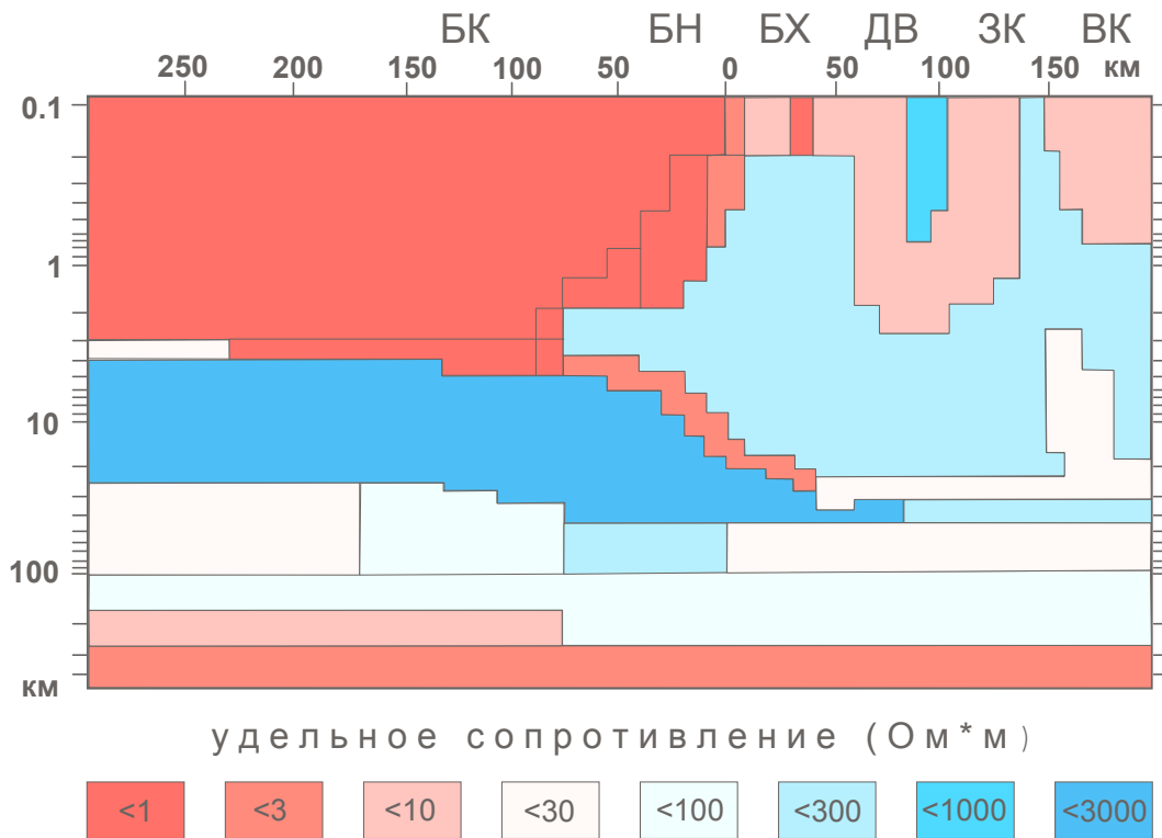
Рис. 11 Двумерная геоэлектрическая модель, полученная И.М.Варенцовым и др. в результате интерпретации данных проекта ЭМСЛАБ (БК – Бассейн Каскадия, БН – Бассейн Ньюпорт, БХ – Береговой Хребет, ДВ – Долина Вилламет, ЗК – Западные Каскады, ВК – Высокие Каскады)
