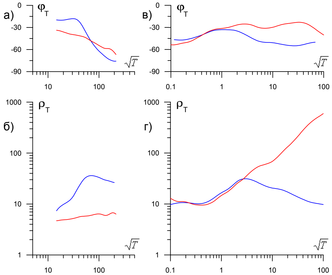
Рис. 9 Типичные кривые МТЗ, полученные в эксперименте ЭМСЛАБ: а), б) донные фазовые и амплитудные кривые (точка наблюдения – в 170 км западнее берега); в), г) наземные фазовые и амплитудные кривые (точка наблюдения – в 48 восточнее от берега). Синие линии – продольные, красные линии – поперечные к берегу и основным структурам кривые
