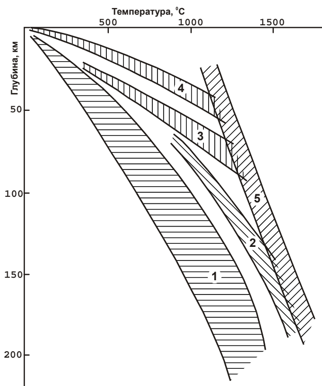
Рис. 2 Геотермы для континентов и океанов: 1 – докембрийские щиты и платформы; 2 – герцениды; 3 – океанские плиты; 4 – альпиды; 5 – солидус сухих пород верхней мантии
