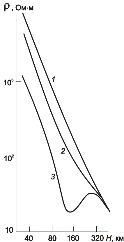
Рис. 7 Прогнозные модели удельного электрического сопротивления континентов для трех различных значений теплового потока: 1 – 40; 2 – 60; 3 – 90 мВт/м 2
