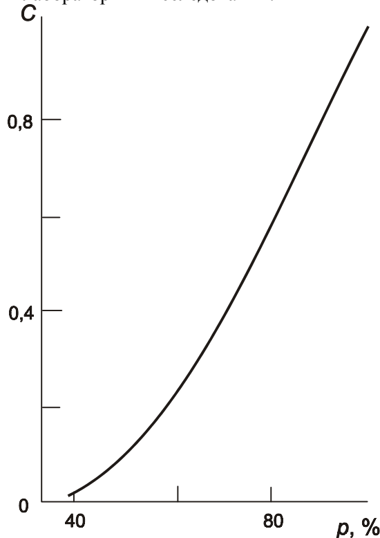
Рис. 3 Зависимость относительной электропроводности от доли связанных каналов
